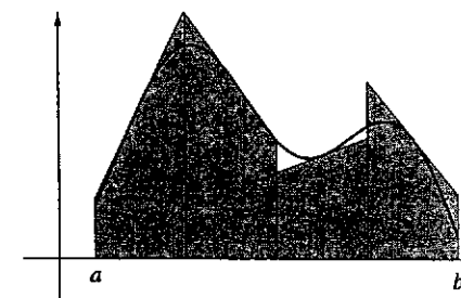
Fig. 10.4 : metodo delle tangenti, n = 4
