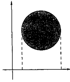
Fig. 8.5 : differenza dei due
