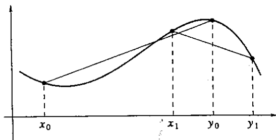
Fig. 6.9 : una funzione continua ma non strettamente monotona
