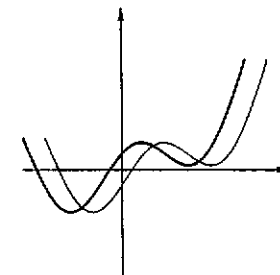
Fig. 4.22 : il grafico di f(x + 1)
