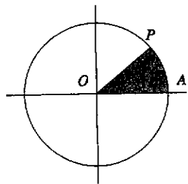
Fig. A4.7: parametrizzazione circolare
