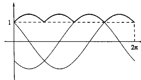
Fig. A9.1 : le funzioni y = \sin(x \pm \frac{\pi}{2}) - \sin x (sottili) e il massimo dei valori assoluti
