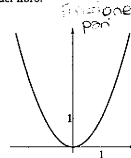
Fig. 1.2: y = x^2
