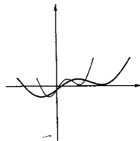
Fig. 4.28 : il grafico di f(x/2)
