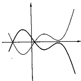
Fig. 4.25 : il grafico di -f(x)
