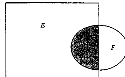
Fig. 2.3 : l'intersezione E \cap F
