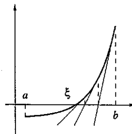
Fig. 10.1 : il metodo di Newton
