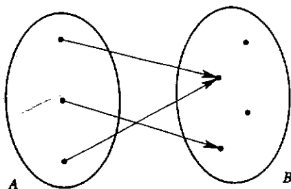
Fig. 2.10 : questa funzione non è iniettiva ...
