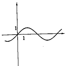
Fig. 1.10 : y = \text{sen } x
