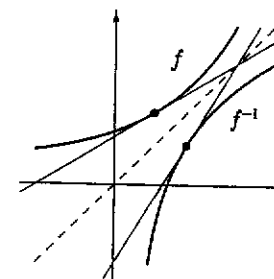
Fig. 7.7 : derivata dell'inversa: interpretazione geometrica
