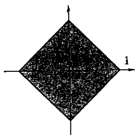
Fig. A4.3: l'insieme B^{(1)}
