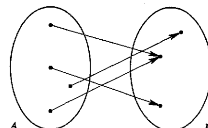
Fig. 2.13 : ... mentre questa è surgettiva
