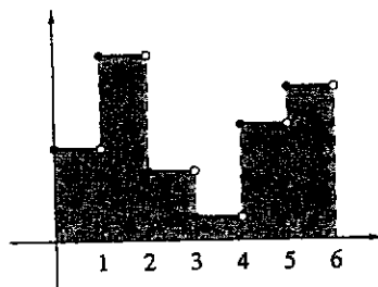
Fig. 8.6 : una somma finita come integrale
