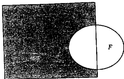
Fig. 2.4 : la differenza E \setminus F ...
