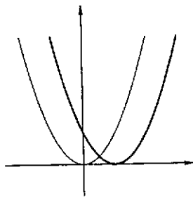
Fig. 4.45 : y = (x-1)^2
