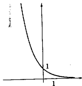
Fig. 1.17 : y = e^{-x}
