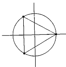
Fig. 3.5 : radici cubiche di 1
