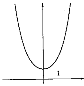
Fig. 4.10: y = \cosh x
