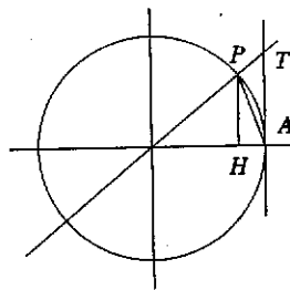
Fig. 4.7: il cerchio goniometrico
