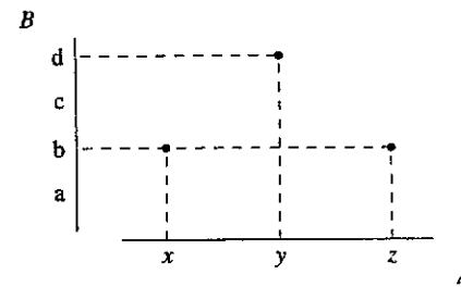
Fig. 2.9 : il grafico della funzione f
