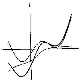
Fig. 4.37 : due funzioni e la loro somma
