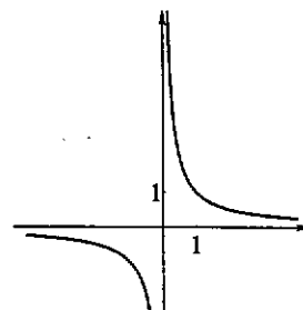
Fig. 6.7 : y = 1/x
