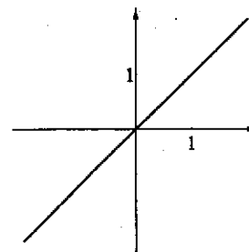
Fig. 1.1: y = x
