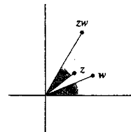
Fig. 3.3 : esempio di prodotto
