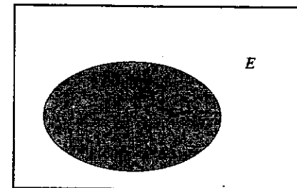
Fig. 2.1 : F è un sottoinsieme di E , cioè F \subset E
