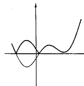
Fig. 4.33 : il grafico di |f(x)|
