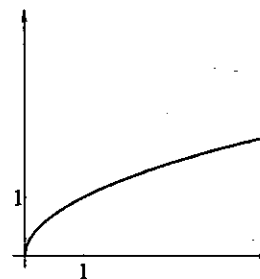
Fig. 1.4: y = \sqrt{x}
