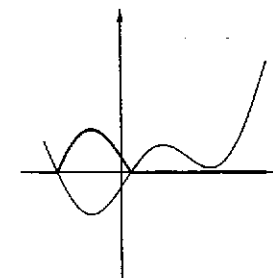
Fig. 4.32 : il grafico di f^-
