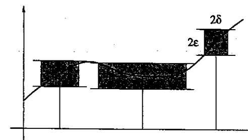
Fig. 6.6 : una funzione continua ( \delta dipende anche da x )
