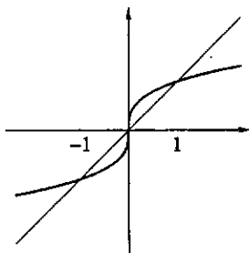
Fig. 5.1 : i grafici di x e \sqrt[3]{x}
