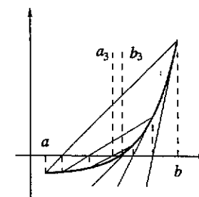
Fig. 10.2 : il metodo delle secanti e tangenti
