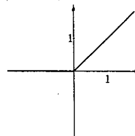
Fig. 4.5 : parte positiva di x
