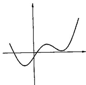
Fig. 4.19 : una generica funzione f
