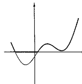
Fig. 4.31 : il grafico di f^+
