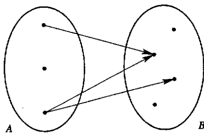
Fig. 2.7 : questa non è una funzione
