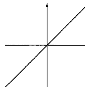
Fig. 2.19 : la relazione R_
