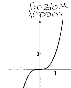
Fig. 1.3: y = x^3
