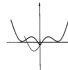
Fig. 4.34 : il grafico di f(|x|)
