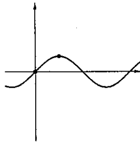
Fig. 4.3 : ... né debolmente decrescente
