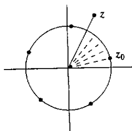
Fig. 3.4 : radici quinte di z
