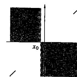
Fig. 7.27 : punto c), limiti di f
