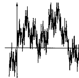
Fig. A9.2 : a = 1.7
