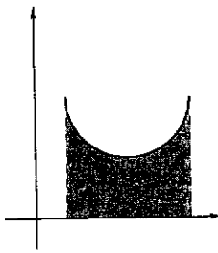
Fig. 8.4 : sottografico di f_2
