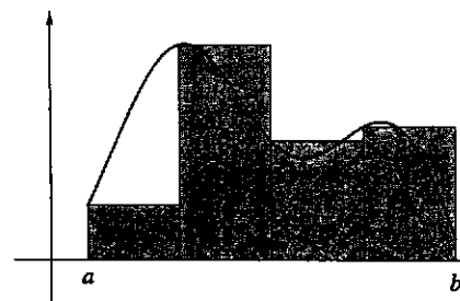
Fig. 10.3 : metodo dei rettangoli, n = 4
