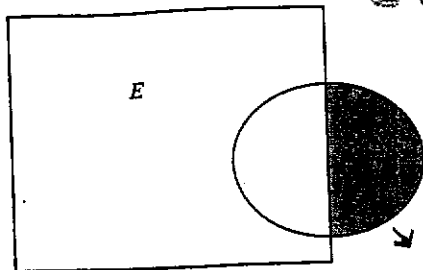
Fig. 2.5 : ... e la differenza F \setminus E
