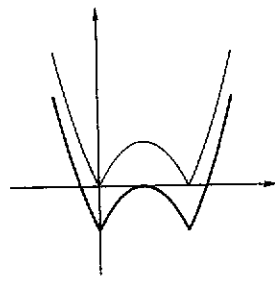
Fig. 4.48 : y = |x^2 - 2x| - 1
