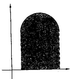
Fig. 8.3 : sottografico di f_1
