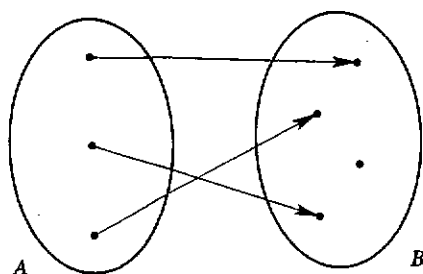
Fig. 2.11 : ... mentre questa è iniettiva
