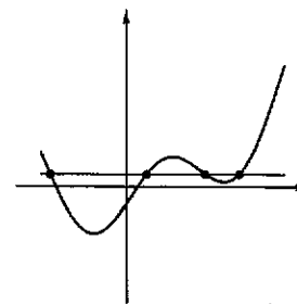
Fig. 4.17 : una funzione non iniettiva
