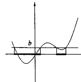
Fig. 4.16 : in neretto la soluzione della disequazione f(x) \leq b
