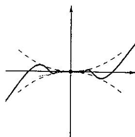
Fig. 7.6 : y = x^2 \sin(1/x)
