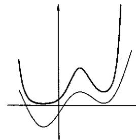
Fig. 4.42 : il grafico di e^{f(x)}
