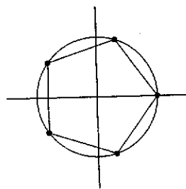
Fig. 3.6 : radici quinte di 1
