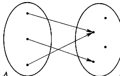
Fig. 2.12 : questa funzione non è surgettiva ...
