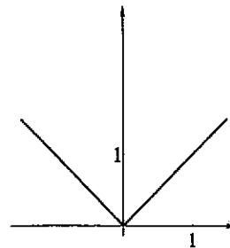
Fig. 4.39 : il grafico di |x|
