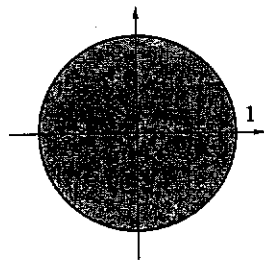
Fig. A4.4: l'insieme B^{(2)}
