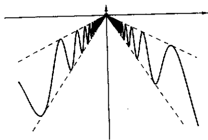
Fig. 7.14 : y = -|x| + \frac{|x|}{2} \sin \frac{1}{x}
