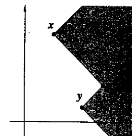
Fig. A2.1 : i maggioranti di x e di y
