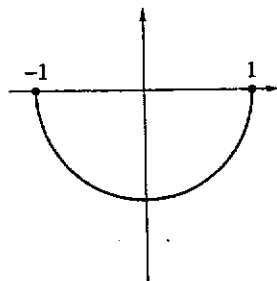
Fig. 7.25 : y = -\sqrt{1-x^2}
