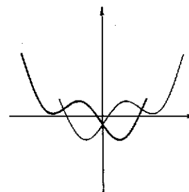
Fig. 4.29 : il grafico di f(-x)
