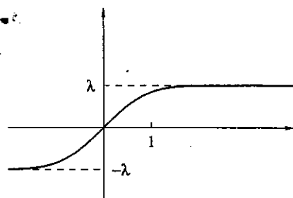
Fig. 8.8 : grafico di \int_0^x e^{-t^2} dt
