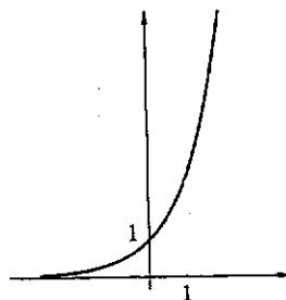
Fig. 1.16 : y = e^x
