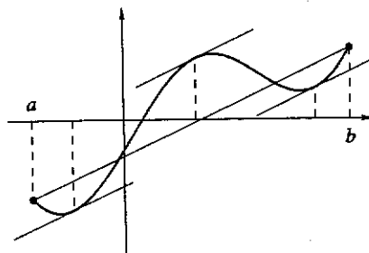
Fig. 7.13 : teorema di Lagrange
