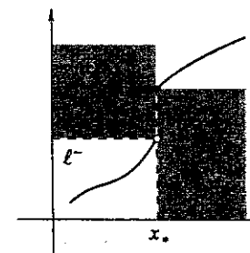
Fig. 6.10 : una funzione monotona e discontinua
