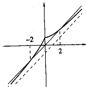
Fig. 7.29 : le intersezioni con y = x
