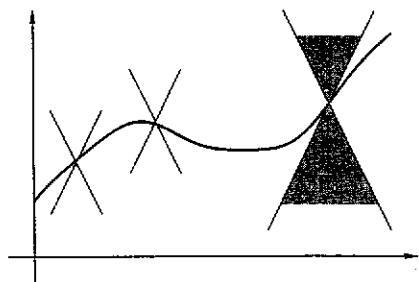
Fig. 6.13 : una funzione lipschitziana
