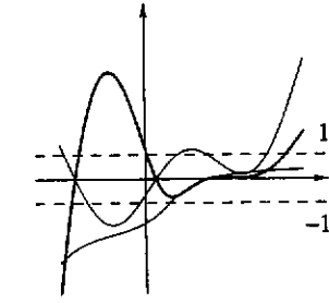
Fig. 4.38 : due funzioni e il loro prodotto
