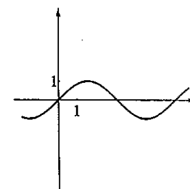
Fig. 7.3 : \sin x è intermedia
