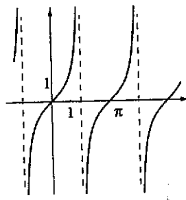
Fig. 1.12 : y = \tan x
