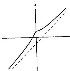
Fig. 7.28 : g) il grafico di f
