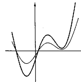
Fig. 4.23 : il grafico di 2f(x)
