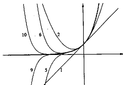
Fig. 7.16 : approssimanti di e^x
