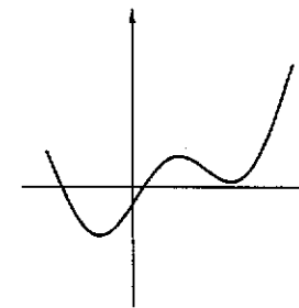
Fig. 4.40 : una funzione f
