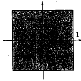
Fig. A4.5: l'insieme B^{(\infty)}
