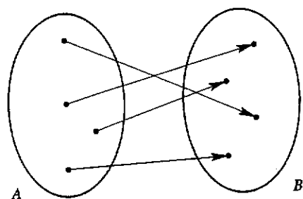
Fig. 2.14 : una funzione biunivoca f: A \rightarrow B
