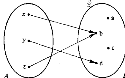
Fig. 2.8 : una funzione f: A \rightarrow B
