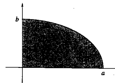
Fig. 8.7 : il sottografico di f(x) = \frac{b}{a} \sqrt{a^2 - x^2} per 0 \leq x \leq a
