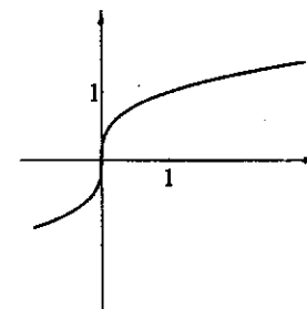
Fig. 1.5: y = \sqrt[3]{x}
