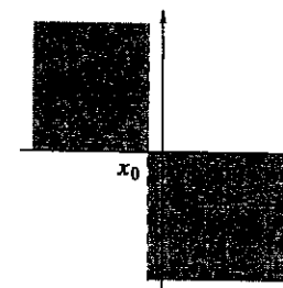
Fig. 7.26 : punto b), segno di f
