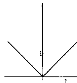
Fig. 1.7: y = |x|
