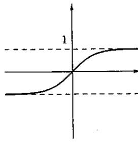
Fig. 4.11: y = \tanh x
