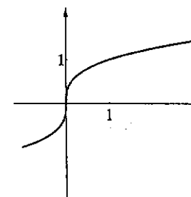
Fig. 7.2 : \sqrt[3]{x} è "ripida"
