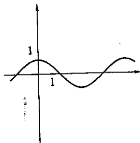
Fig. 1.11 : y = \cos x
