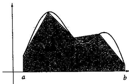
Fig. 10.5 : metodo dei trapezi, n = 4
