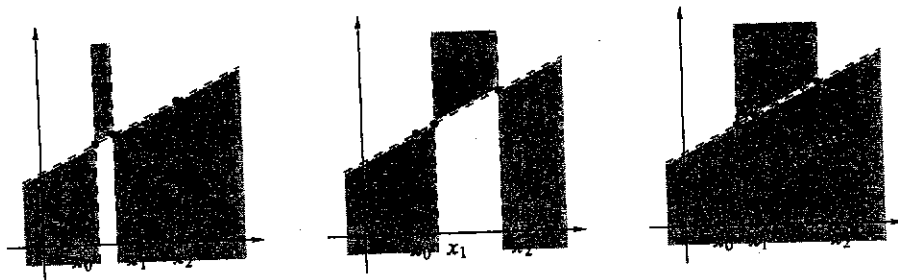
Fig. 7.22 : unione delle due
