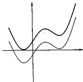
Fig. 4.20 : il grafico di f(x) + 2
