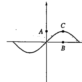
Fig. 4.1 : valore massimo, punto di massimo, punto sul grafico
