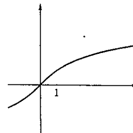
Fig. 4.12: y = \text{settsinh } x
