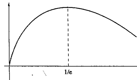
Fig. A6.1 : il grafico di f(x) = -x \log x
