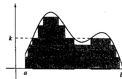
Fig. A8.1 : in neretto l'insieme dove f(x) \geq k
