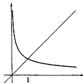
Fig. 5.2 : i grafici di x e 1/\sqrt{x}
