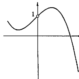
Fig. 6.2: f non è definita in x=0
