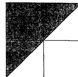
Fig. 2.20 : la relazione R_ \leq
