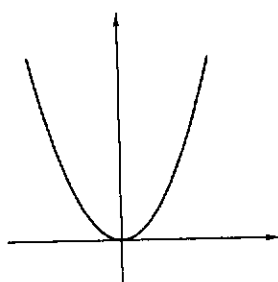
Fig. 4.44 : y = x^2
