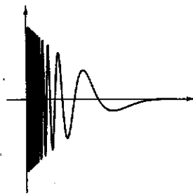
Fig. 6.12 : y = (1 - \frac{x}{2})^2 \sin \frac{6}{x} su ]0, 2]
