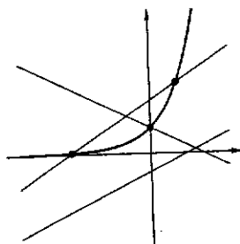
Fig. 7.23 : nessuna, una, due intersezioni
