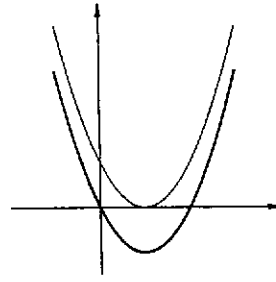
Fig. 4.46 : y = (x-1)^2 - 1
