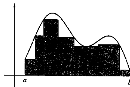
Fig. 8.1 : plurirettangolo inscritto ...
