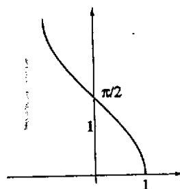
Fig. 1.14 : y = \arccos x
