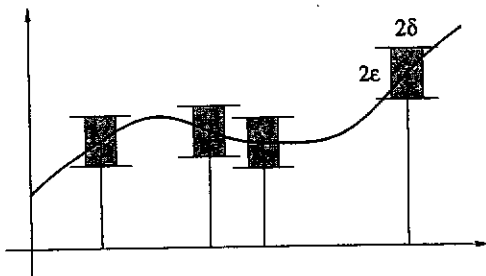
Fig. 6.14 : questo valore di \delta è adatto in ogni punto
