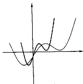
Fig. 4.27 : il grafico di f(2x)
