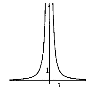
Fig. 1.9: y = 1/x^2
