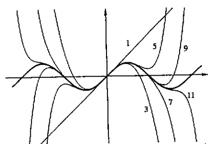
Fig. 7.15 : approssimanti di \sin x
