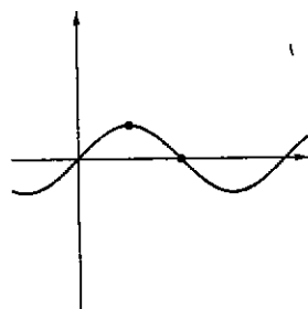
Fig. 4.2 : \sin x non è debolmente crescente ...
