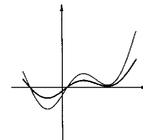
Fig. 4.24 : il grafico di f(x)/2
