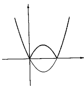
Fig. 4.47 : y = |x^2 - 2x|
